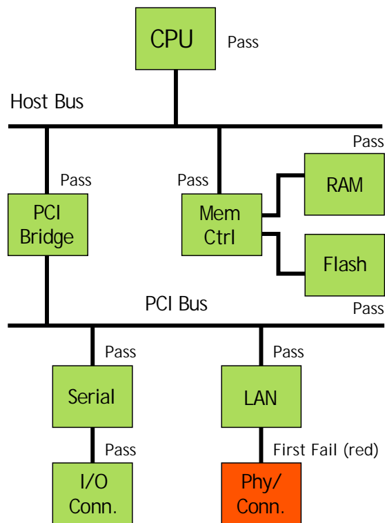
Fig. 7 – LAN Port failure.
